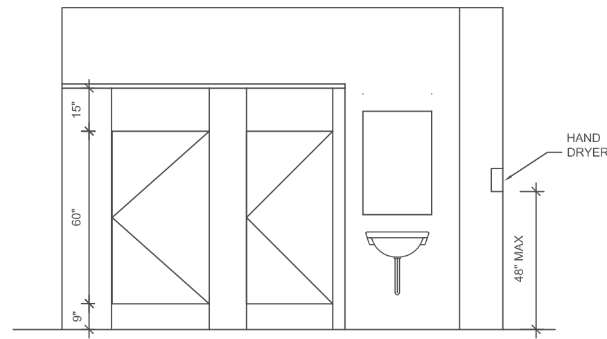
ELEVATION - 2
